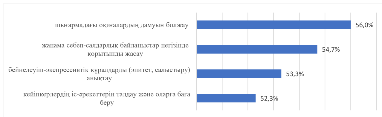
3-сурет. 9-сынып білім алушыларының оқу сауаттылығы бойынша ББЖМ нәтижелері
